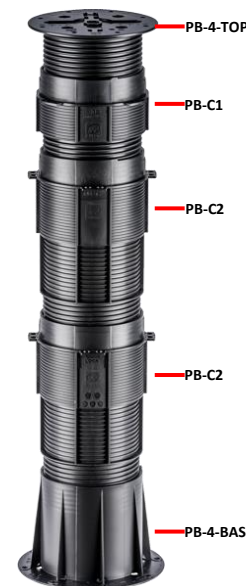
PB-10 675-830 мм
