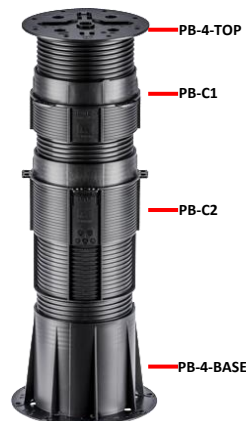
PB-8 480-595 мм
